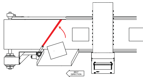
DIVERT ARM
